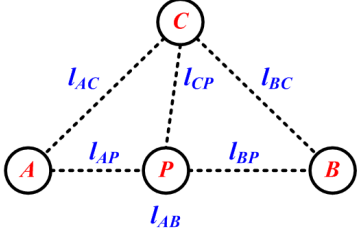
Fig. 1. Illustration of Lemma 1
